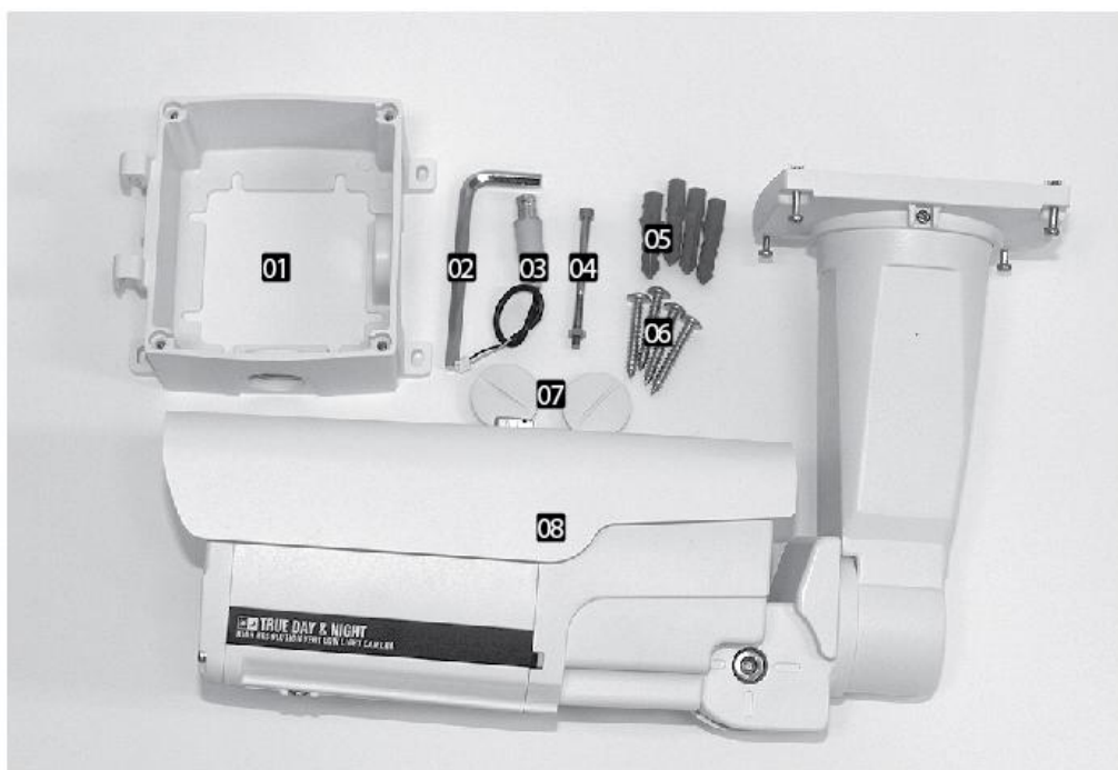
1. Монтажный корпус 2. Ключ 3. Дополнительный видеокабель 4. Соединительный винт монтажной коробки 5. Анкеры 4шт. 6. Винты 4 шт. 7. Крышки 2шт. 8. Камера
