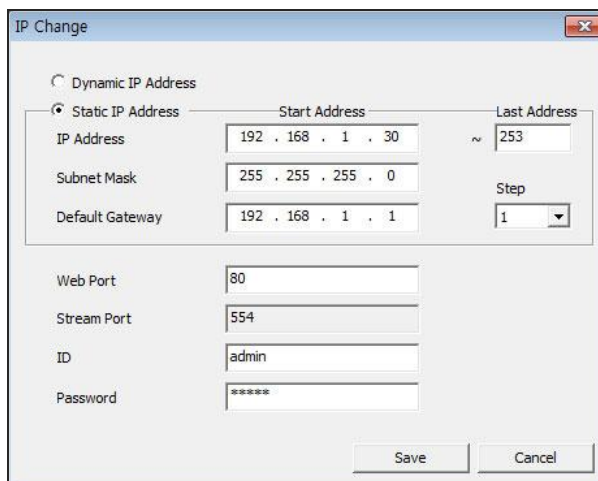
[Рис. 5-5] Диалоговое окно изменения IP-адреса
