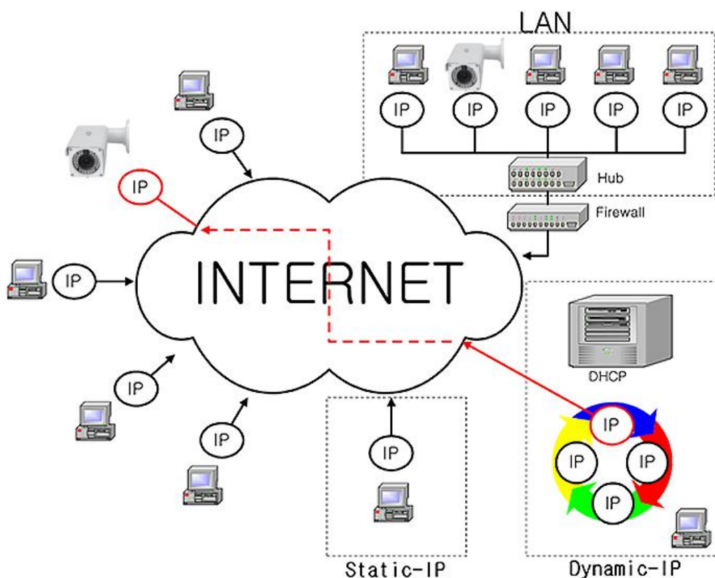
[Рис. 6-1] Интернет-среда
