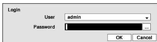
Рисунок 5. Экран регистрации.
