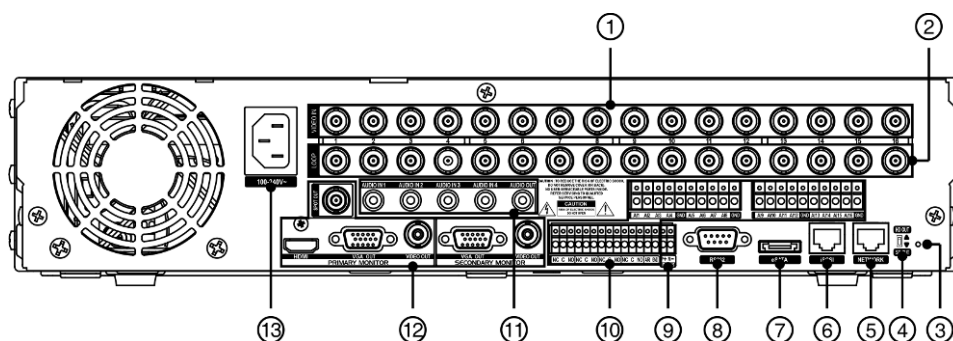
Рисунок 2. Задняя панель 16-канальной модели цифрового видеорегистратора.
