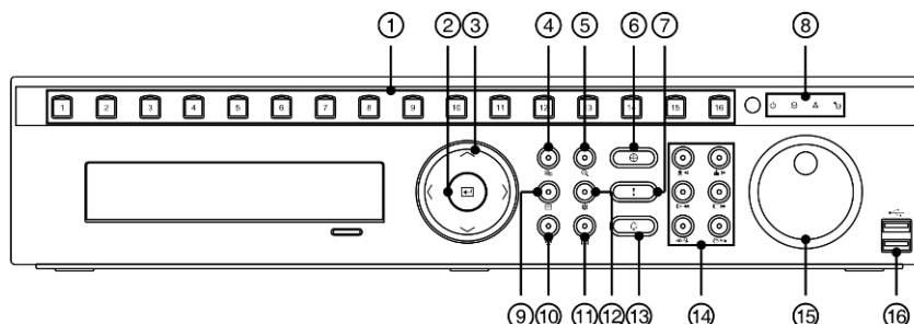
Рисунок 3. Передняя панель 16-канальной модели цифрового видеорегистратора.
