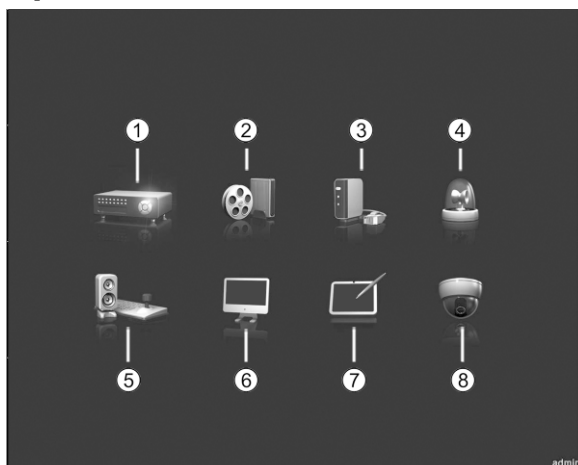
Рисунок 7. Экран настройки.
